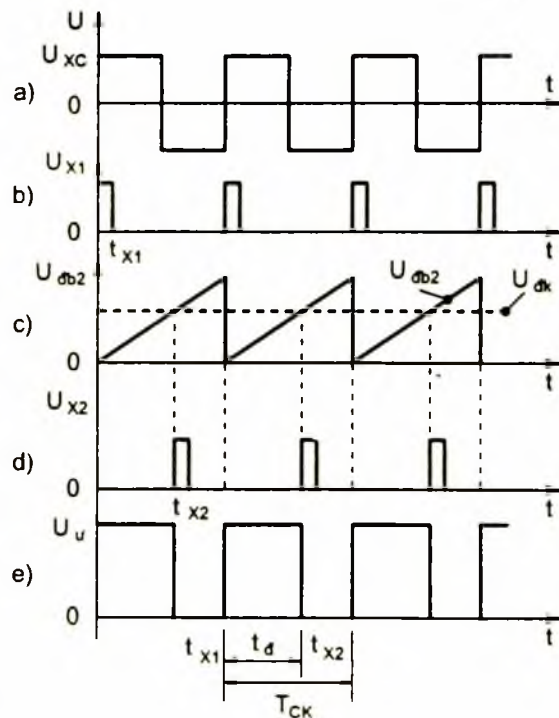
Hình 4 - 19. a,b,c,d) Dạng xung điện áp trên đầu ra của các khâu trong mạch điều khiển ; e) Dạng điện áp đặt lên phản ứng động cơ
