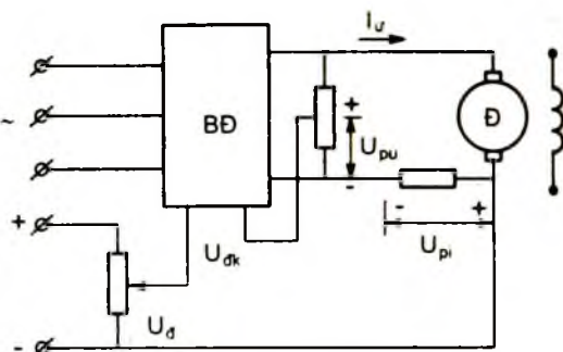
Hình 3 - 31. Sơ đồ nguyên lý hệ Bộ biến đổi - Động cơ có phản hồi hỗn hợp
