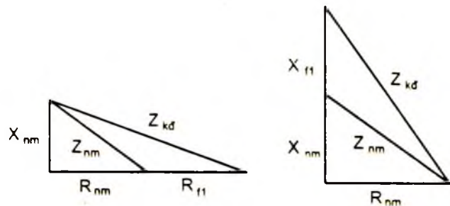
Hình 3 - 18. Tam giác tổng trở
