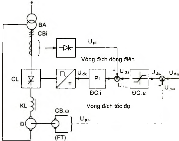
13b. Sơ đồ nguyên lý hệ CL - Đ tự động có điều chỉnh tốc độ kiểu nối tiếp
