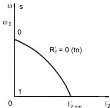
Hình 2 - 24. Đặc tính cơ điện vẽ theo dòng roto của động cơ không đồng bộ
