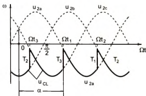
Hình 4 - 6. Đồ thị điện áp (sdd) của bộ chỉnh lưu ở trạng thái nghịch lưu
