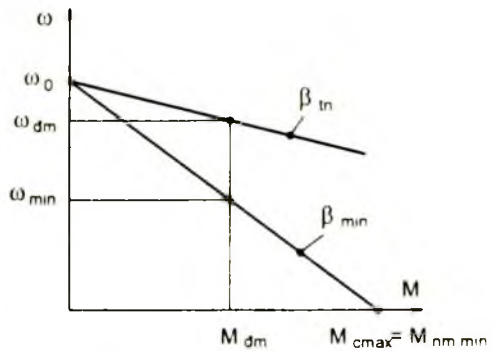
Hình 3 - 4. Giải thích về dải điều chỉnh tốc độ theo khả năng quá tải yêu cầu
