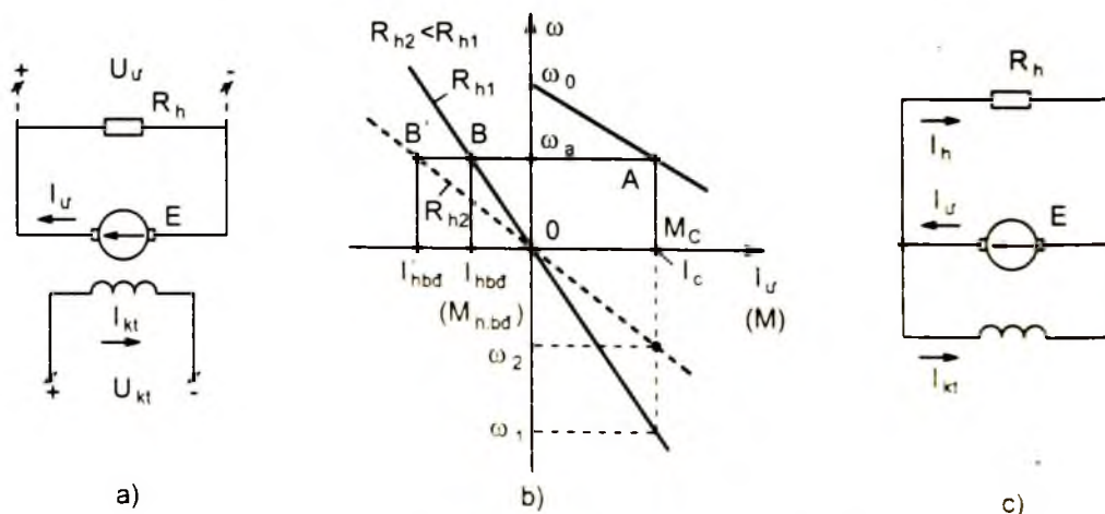
Hình 2 - 11 a) Sơ đồ nối dây hãm động năng kích từ độc lập b) Đặc tính cơ hãm động năng kích từ độc lập : c) Sơ đồ hãm động năng tự kích
