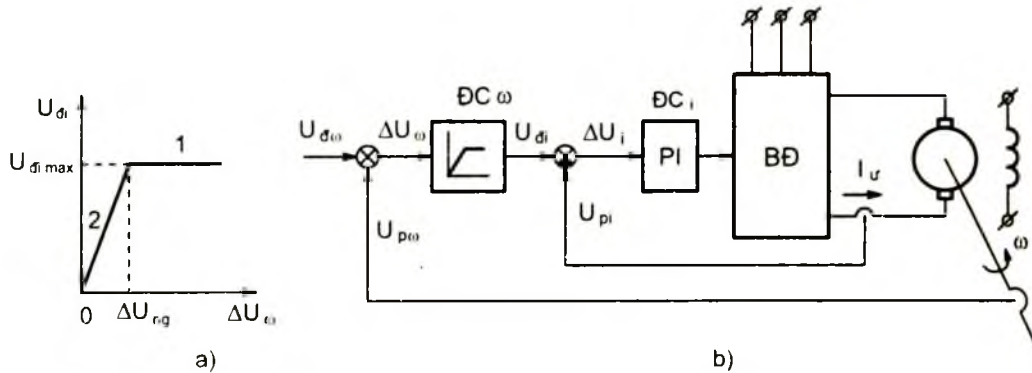
Hình 3 - 33. Nguyên tắc hạn chế dòng điện và momen nhờ khâu hạn chế ở đầu vào a) Đặc tính khâu hạn chế ; b) Sơ đồ nguyên lý toàn hệ thống
