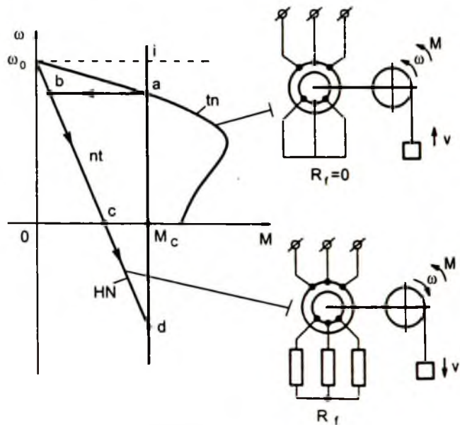
Hình 2 - 33. Hãm ngược nhờ tải trọng (hạ tải) thực hiện bằng cách nối điện trở phụ vào mạch roto (đoạn cd) dùng cho động cơ roto dây quấn
