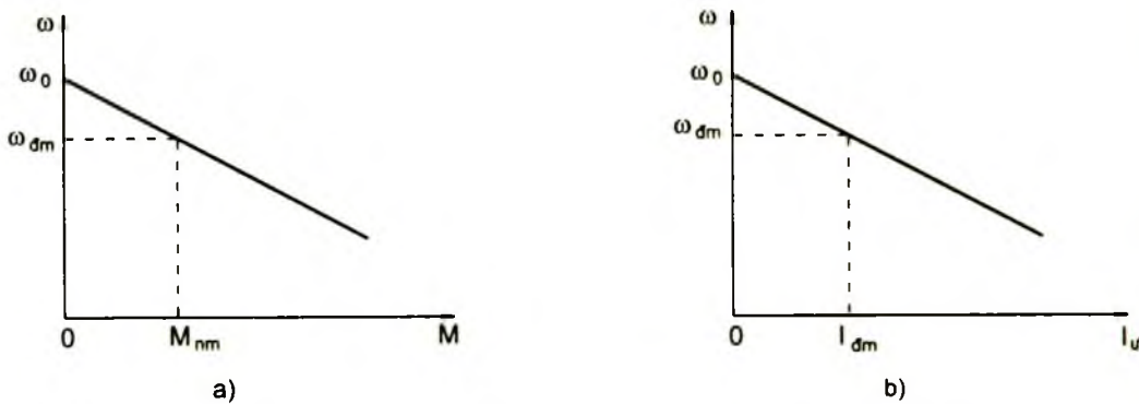
Hình 2 - 3. a) Đặc tính cơ tự nhiên của động cơ điện một chiều kích từ độc lập :
