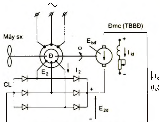
Hình 4 - 27. Sơ đồ nguyên lý tăng điện cơ
