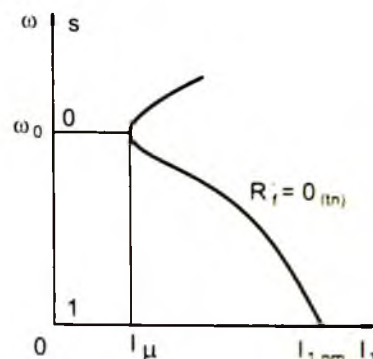
Hình 2 - 25. Đặc tính cơ điện vẽ theo dòng stato của động cơ không đồng bộ
