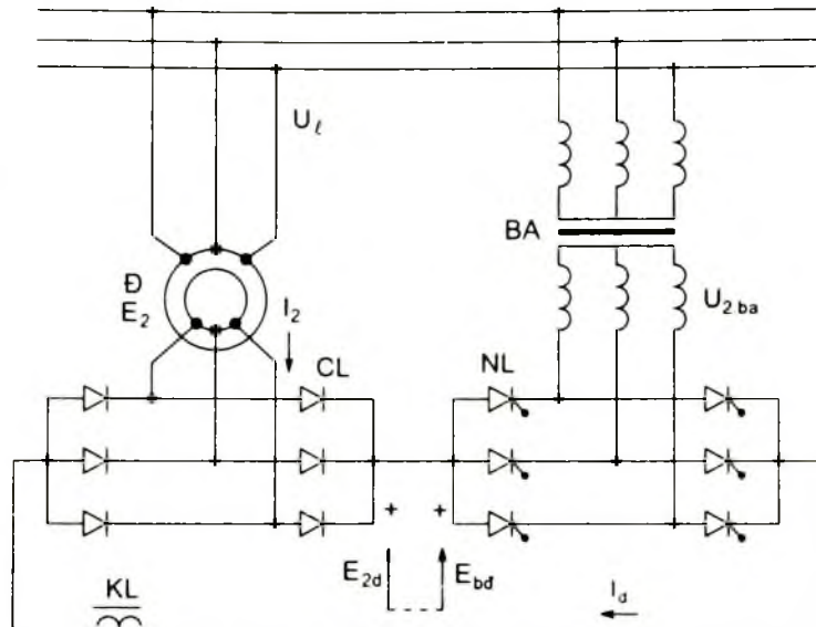
Hình 4 - 28. Sơ đồ tầng điện
