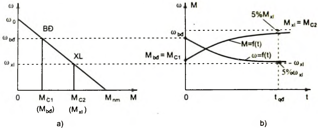
Hình 5-1. Các đặc tính quá độ M = f(t) và \omega = f(t) của quá trình quá độ cơ học
