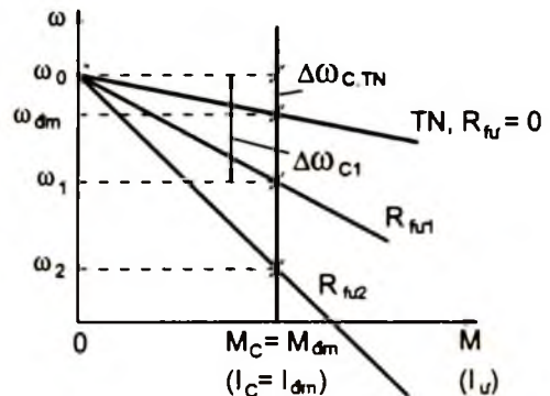
Hình 2 - 4. Họ đặc tính nhân tạo biến trở
