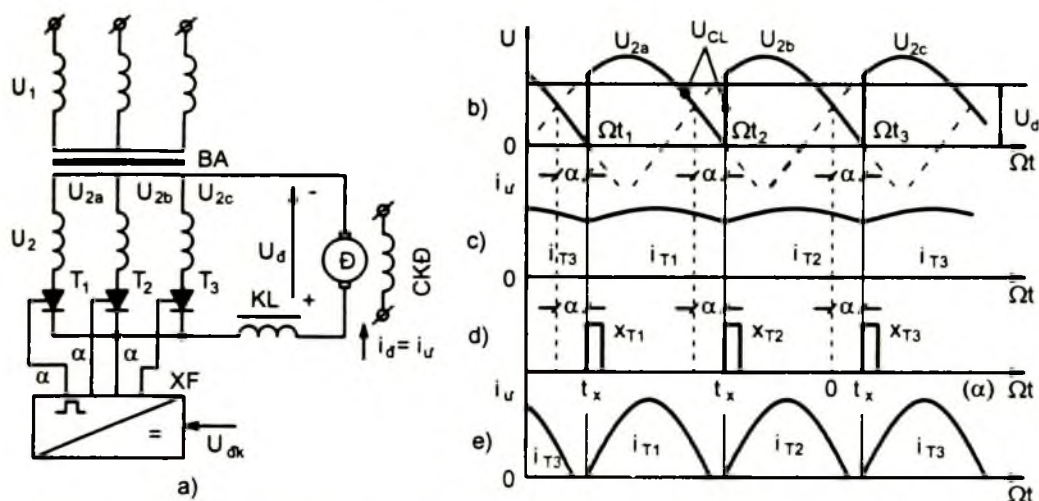
Hình 4 - 3. Sơ đồ nguyên lý (a) và các đồ thị điện áp, dòng điện (b, c, e) và xung mở van (d) của hệ CL-Đ không đảo chiều
