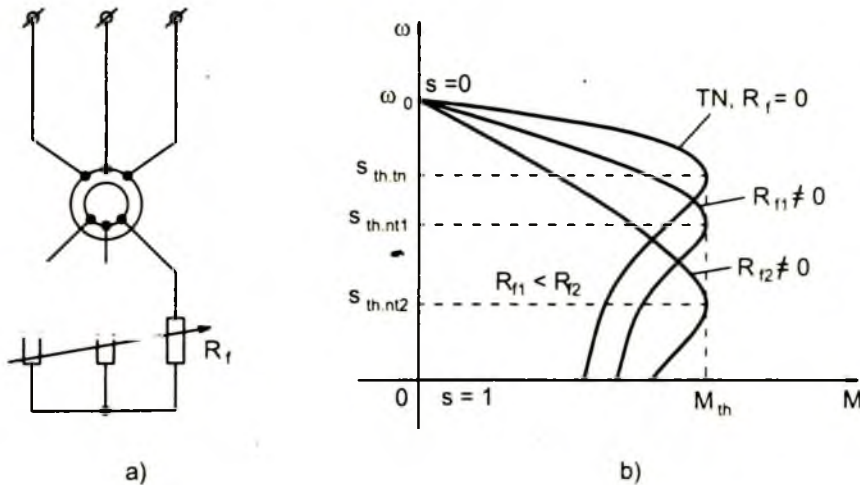
Hình 2 - 27. Sơ đồ nối dây (a) và họ đặc tính cơ nhân tạo khi thay đổi điện trở mạch roto(b) của động cơ không đồng bộ
