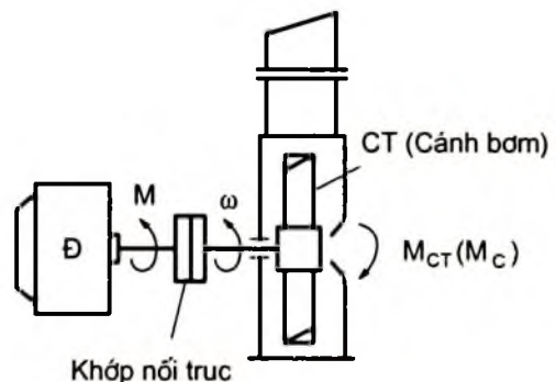
Hình 1 -1. Truyền động của máy bơm nước
