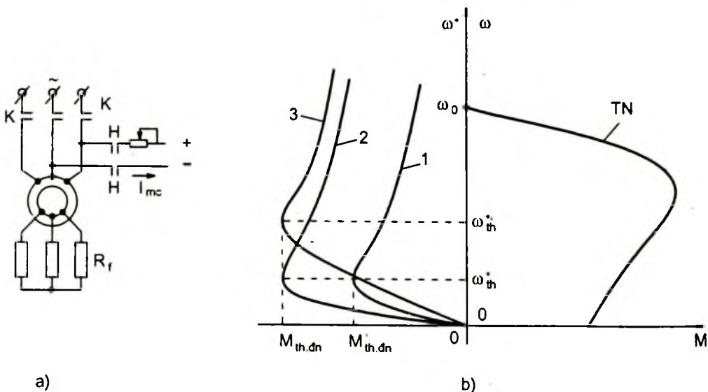
Hình 2 - 35. Hãm động năng động cơ không đồng bộ. a) Sơ đồ nguyên lý :
