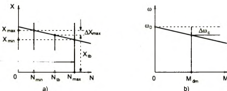
Hình 3 - 1. Cách xác định S%
