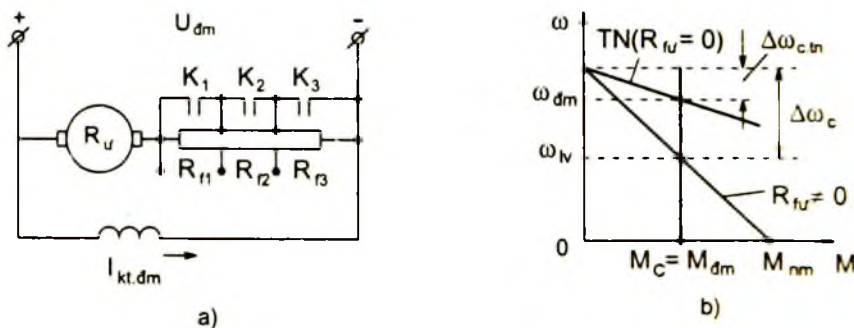
Hình 3 - 3. Điều khiển động cơ một chiều kích từ song song bằng phương pháp dùng điện trở phụ mạch phản ứng
