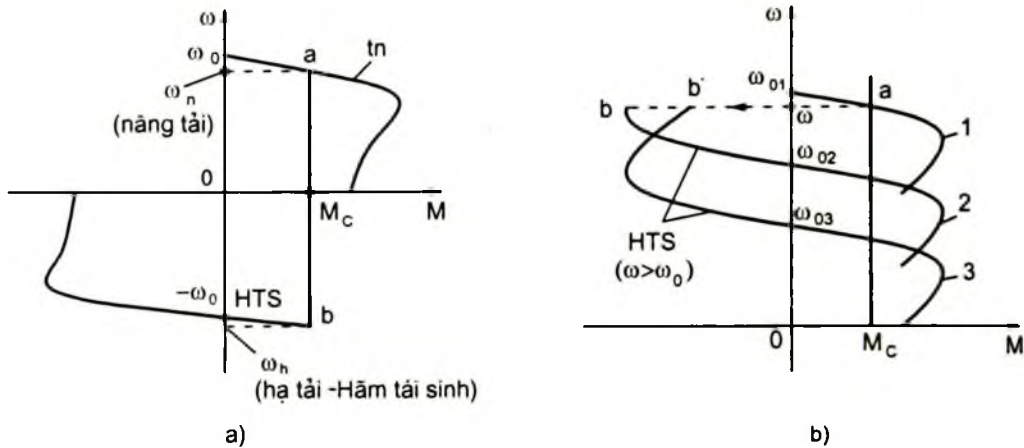
Hình 2 - 32. Các đặc tính cơ của động cơ không đồng bộ khi hãm tái sinh
