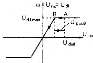
Hình 4 - 14. Đặc tính của bộ điều chỉnh tốc độ ĐC \omega
