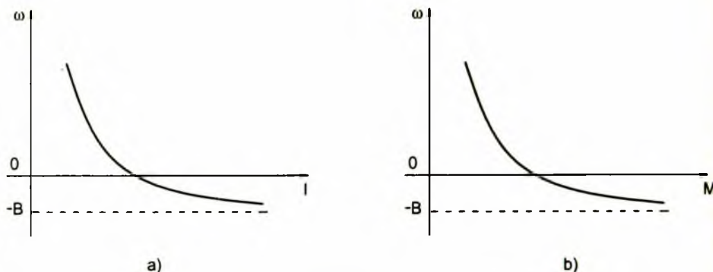
Hình 2 - 14. a) Đặc tính cơ điện của động cơ một chiều kích từ nối tiếp; b) Đặc tính cơ của động cơ một chiều kích từ nối tiếp.
