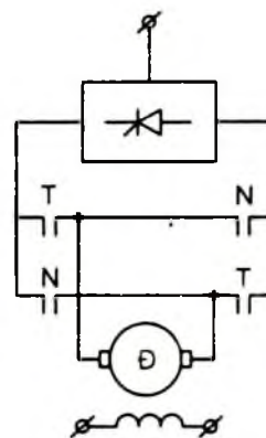
Hình 4 - 9. Sơ đồ nguyên lý hệ CL - Đ đảo chiều dùng bộ tiếp điểm thuận nghịch trong mạch phản ứng
