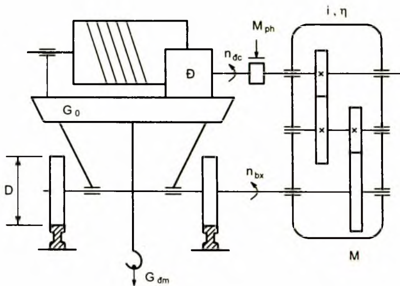
Hình 6 - 7. Kết cấu cơ khí của xe trục
