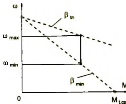
Hình 3 - 5. Đặc tính momen tải cho phép của động cơ một chiều khi điều chỉnh bằng điện trở phụ trong mạch phản ứng
