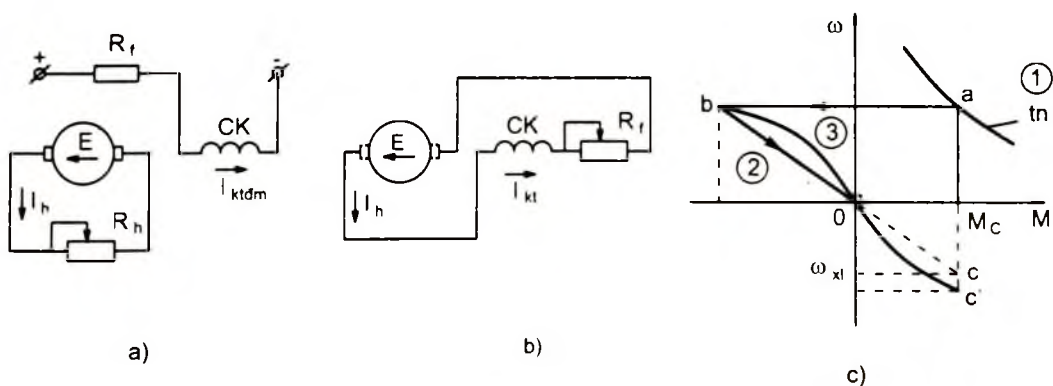
Hình 2 - 19. Hãm động năng động cơ một chiều kích từ nối tiếp
