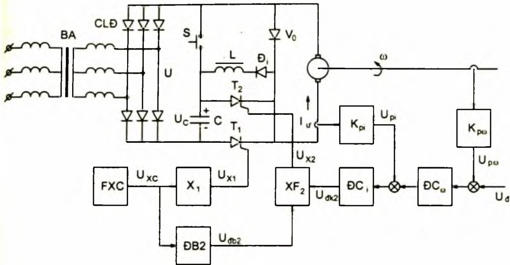
Nguyên lý hệ DAX - D có khoá tiristo và điều chỉnh độ rộng xung
