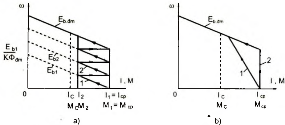
Hình 3 - 12. Điều chỉnh dòng điện và momen của động cơ một chiều bằng cách thay đổi điện áp phản ứng
