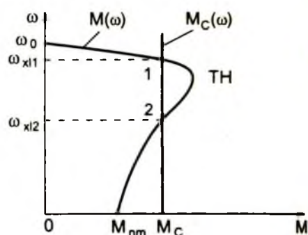
Hình 1 - 13. Điểm làm việc ổn định (1) và không ổn định (2)
