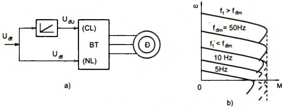
hối và đặc tính cơ của hệ BT - Đ điều khiển theo luật U/f = \text{const}
