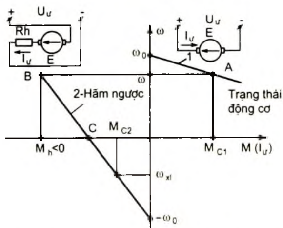
Hình 2 - 10. Hãm ngược khi đảo cực tính điện áp nguồn U_d
