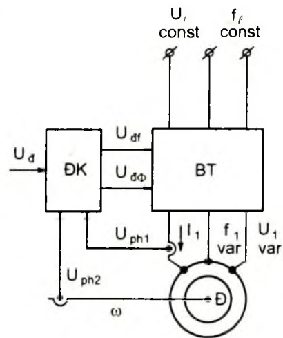
Hình 3 - 19. Sơ đồ khái quát hệ BT - Đ
