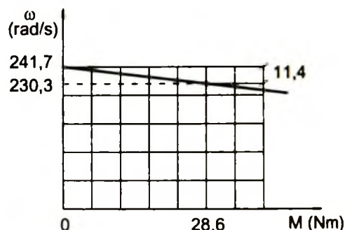
Hình 2 - 7. Đặc tính cơ tự nhiên của động cơ trong ví dụ 2 - 1.
