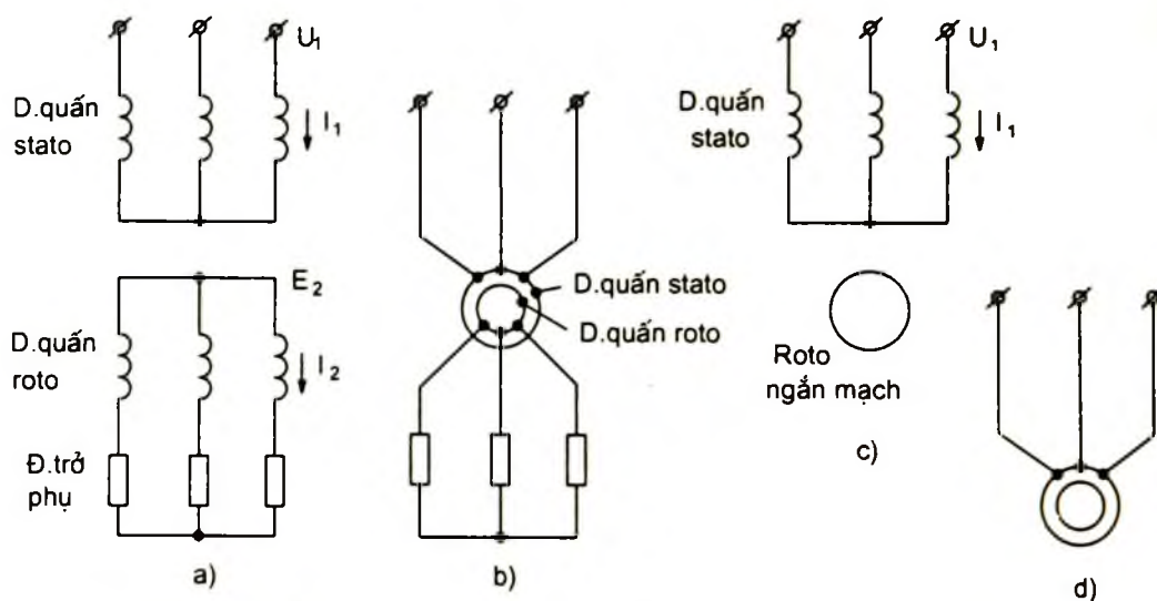
Hình 2 - 22. Sơ đồ nối dây và ký hiệu bản vẽ của động cơ không đồng bộ vẽ cho trường hợp dây quấn stato nối Y)
