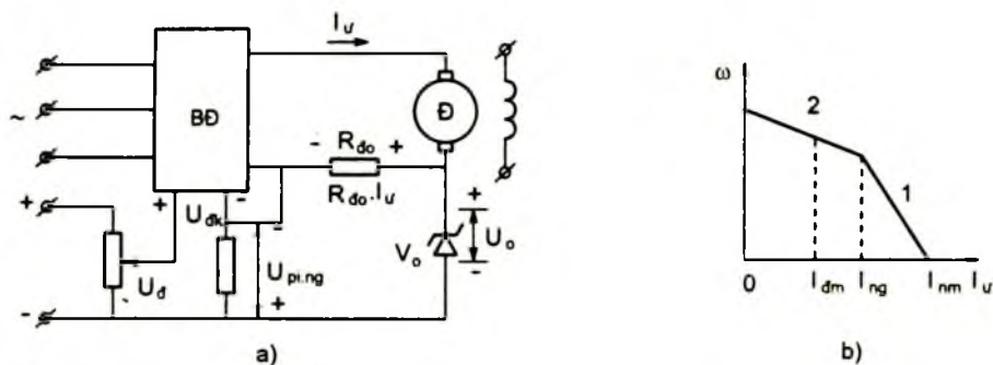
Hình 3 - 32. a) Sơ đồ nguyên lý hệ BĐ - Đ có phản hồi âm dòng điện có ngắt ; b) Đặc tính máy xúc
