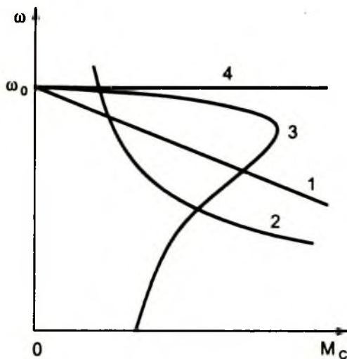
Hình 1 - 10. Đặc tính cơ của các động cơ điện
