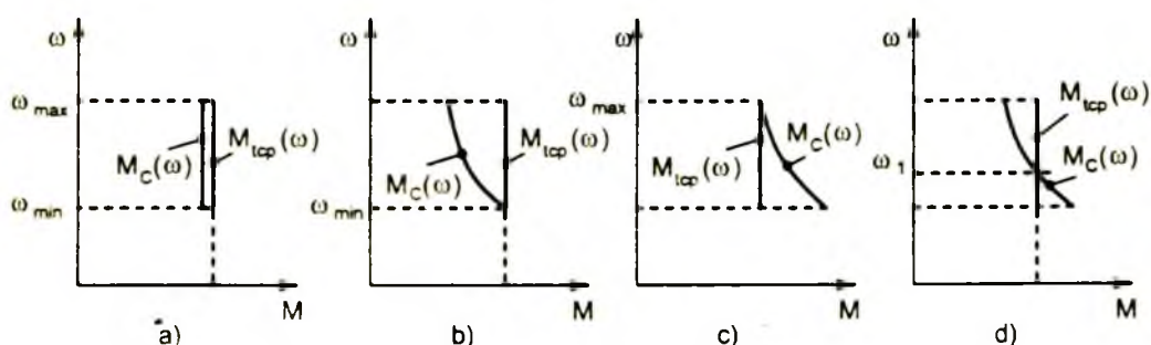
h 6 - 10. So sánh đặc tính tải cho phép của động cơ ( M_{t_{cp}} ) và đặc tính cơ của máy sản xuất ( M_c )
