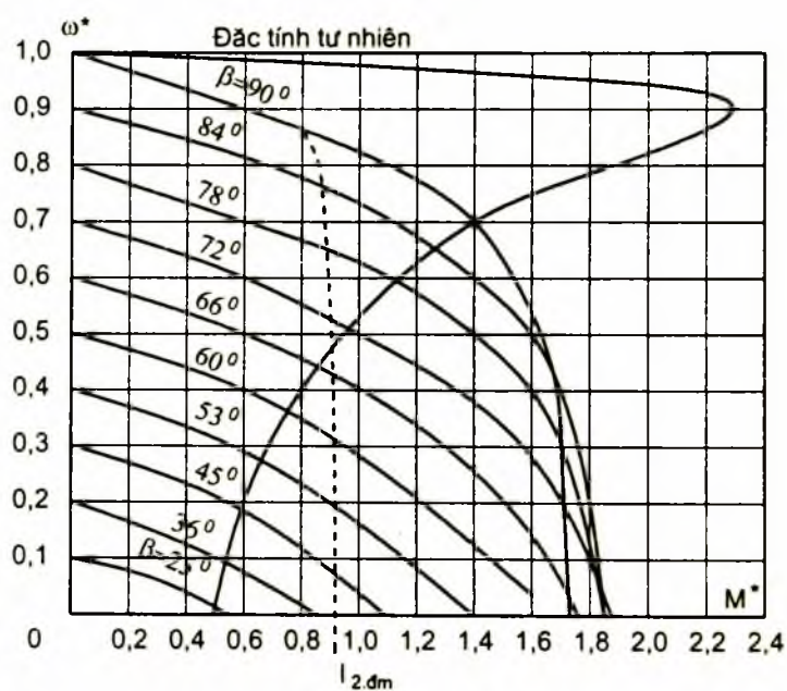
Hình 4 - 29. Họ đặc tính cơ của động cơ 100kW - 1450vg/ph - 380V nối theo sơ đồ tăng điện
