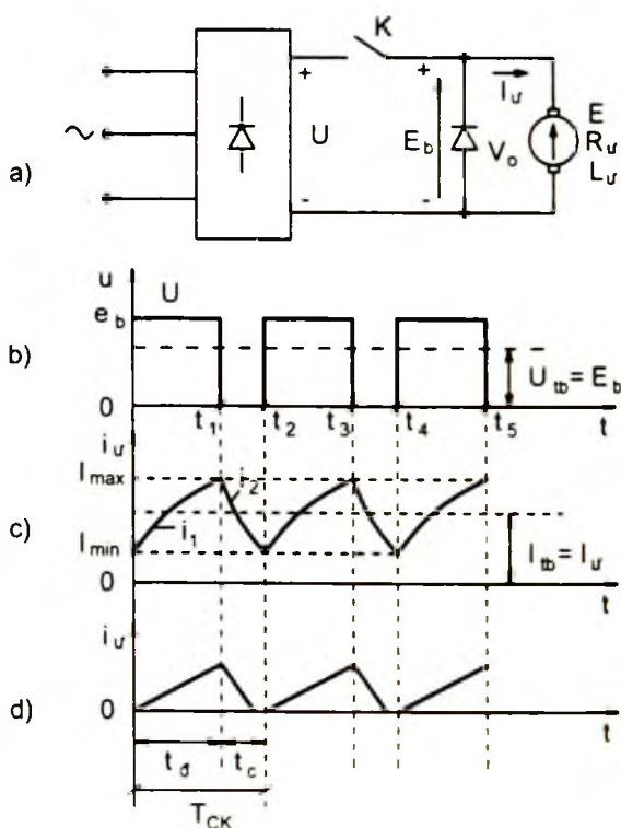
Hình 4 - 16. a) Sơ đồ nguyên lý hệ ĐAX - Đ;
