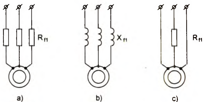
Hình 3 - 17. Các sơ đồ nối điện trở - điện kháng phụ để khởi động động cơ lồng sóc
