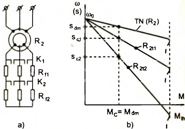
Hình 3 -13. Điều khiển động cơ không đồng bộ roto dây quấn bằng điện trở phụ trong mạch roto
