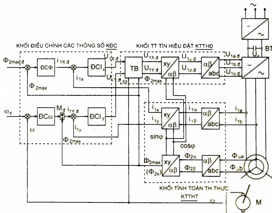
Hình 4 - 25. Sơ đồ khối (nguyên lý) của hệ BT-DKDB có điều khiển vector duy trì từ thông \Phi_{2\max} và dùng cảm biến từ thông (Hệ thống Transvector)
