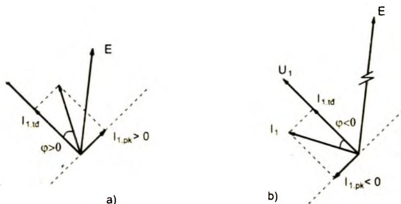
Hình 3 - 26. a) Đồ thị vectơ của động cơ đồng bộ trong trường hợp thiếu kích từ ; b) Đồ thị vectơ của động cơ đồng bộ trong trường hợp quá kích từ
