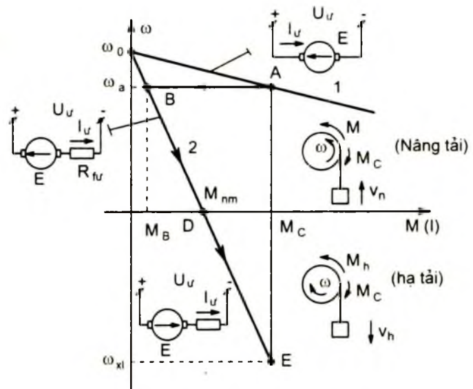
Hình 2 - 9. Hãm ngược khi hạ tải trọng
