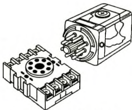
Hình 9-2. Rơ-le điều khiển.
