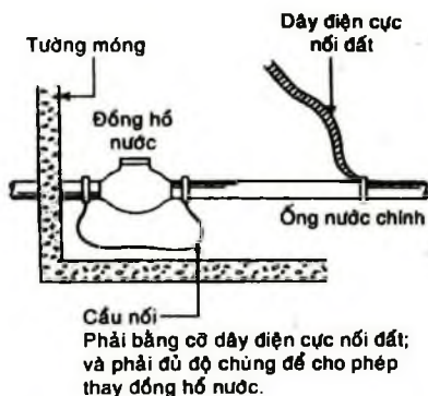
Hình 8-6. Cách liên kết xung quanh đồng hồ nước.
