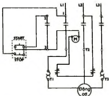
Hình 3-6. Sơ đồ đấu nối bộ khởi động từ của động cơ.
