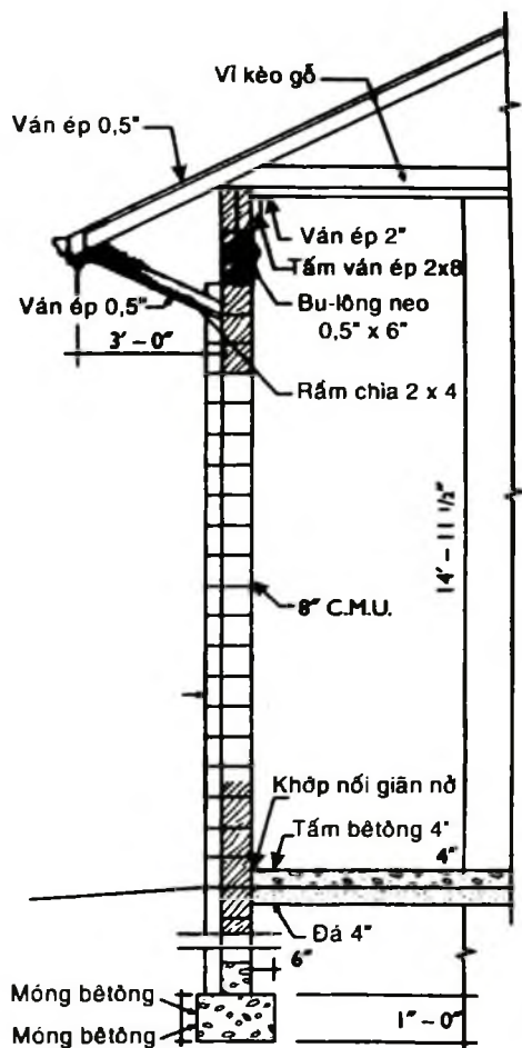
Mặt cắt tường
