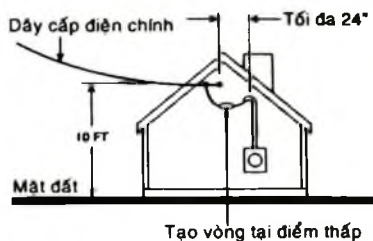
Hình 7-7. Vòng nhỏ giọt
