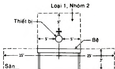
Hình 14-20. Các vị trí Loại 1.
