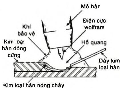
Hình 10-7. Hàn TIG
