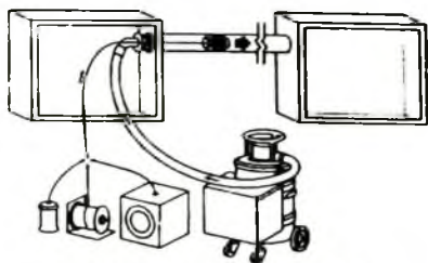
Hình 12-13. Hệ thống thối.
