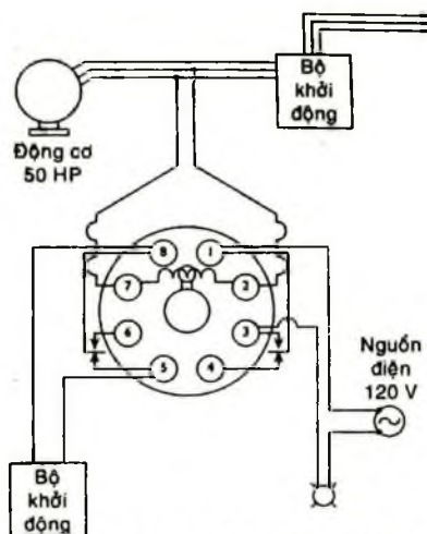
Hình 9-4. Rơ-le tám chân trong mạch điện.
