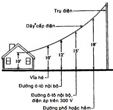
Hình 7-2. Chiều cao dây cáp điện chính.
