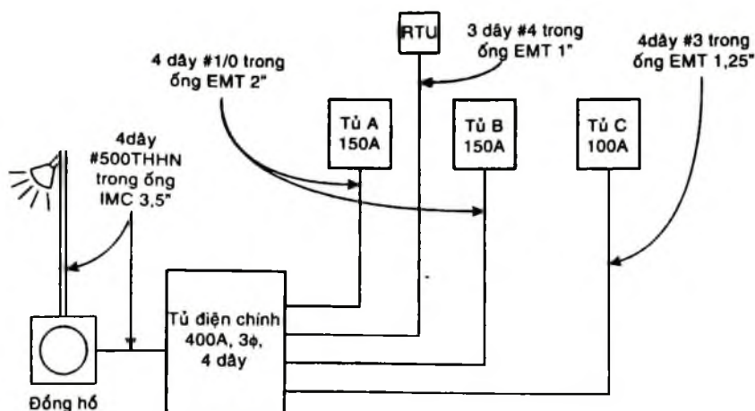
Hình 7-1. Hệ thống phân phối điện.
