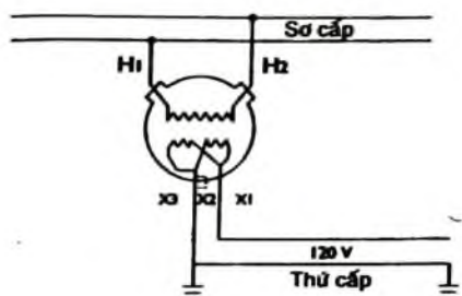
Hình 11-4. Nối kết biến áp một pha, 120 volt.
