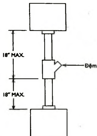
Hình 14-1. Bố trí chất làm kín trên đường dây ngấn.
