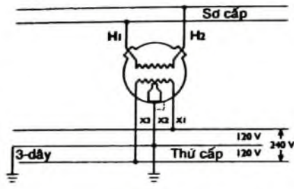
Hình 11-5. Nối kết biến áp một pha, 120/240 V
