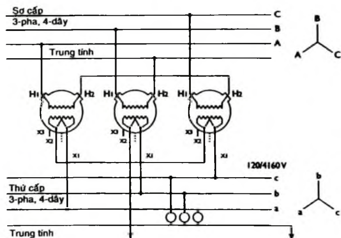
Hình 11-12. Đấu sao-sao
