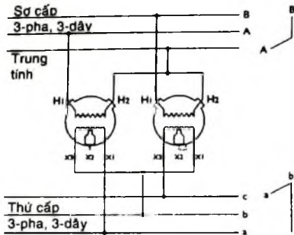
Hình 11-10. Đấu sao-tam giác hở
