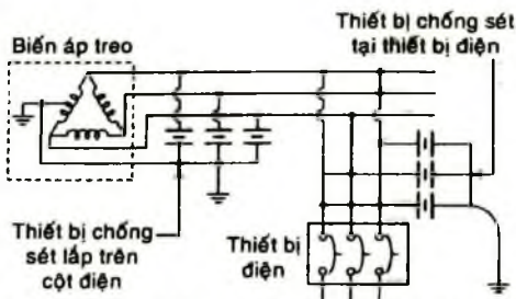
Hình 8-13. Cách nối kết thiết bị chống sét lan truyền.
