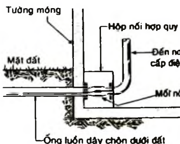
Hình 7-6. Cách nối các dây cáp điện chính đi ngầm dưới đất.
