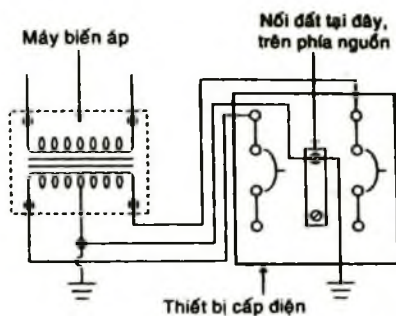
Hình 8-2. Nối đất hệ thống cấp điện
