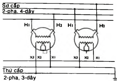
Hình 11-7. Nối kết máy biến áp 2-pha.
