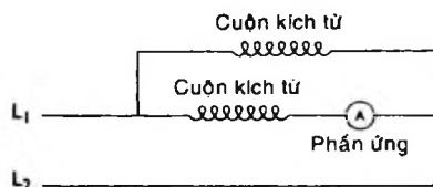
Hình 4-8. Động cơ dc hỗn hợp
