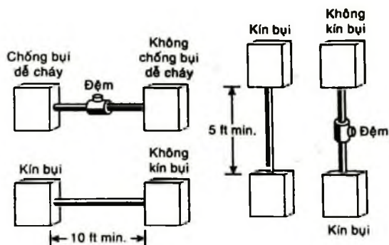
Hình 14-6. Các quy định làm kín.
