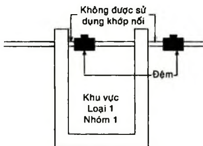
Hình 14-3. Các đệm kín dùng cho khu vực Loại 1, Nhóm 1.
