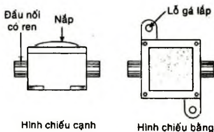
Hình 14-5. Hộp chống nổ
