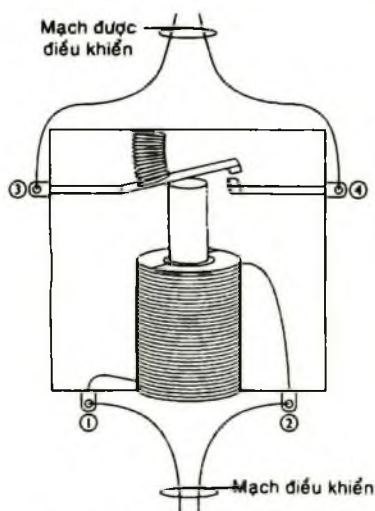
Hình 9-1. Rơ-le căn bản.
