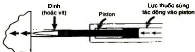
Hình 15-5. Nguyên lý tác động gián tiếp.
