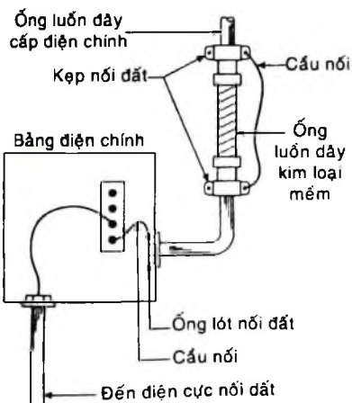
Hình 7-11. Nối kết xung quanh ống luồn dây cấp điện chính
