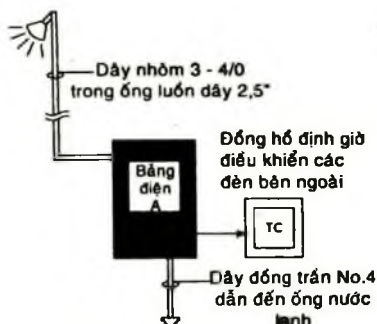
Hình 3-4. Sơ đồ cấp điện
