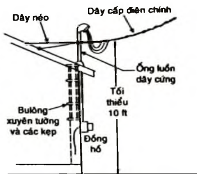
Hình 7-5. Đồ gá trụ đỡ dây cáp điện chính
