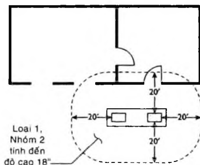
Hình 14-12. Các vị trí Loại 1, Nhóm 2.
