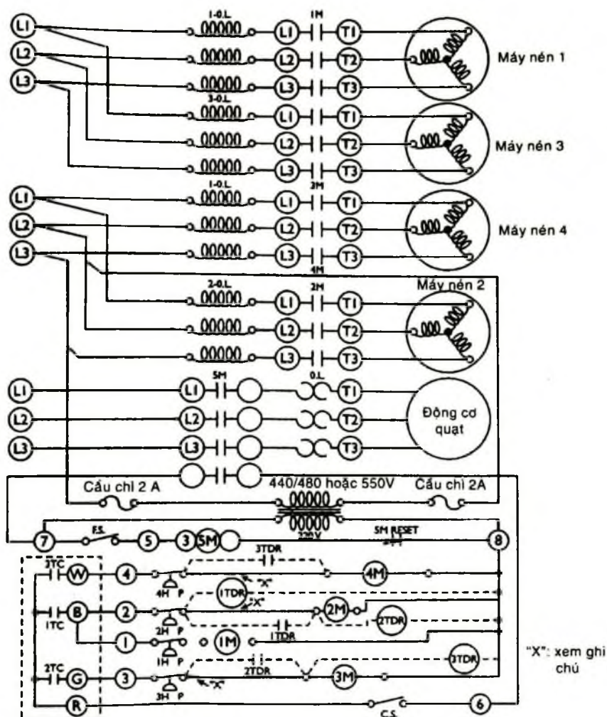
Hình 3-5. Sơ đồ đi dây.
