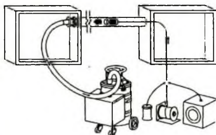
Hình 12-12. Hệ thống hút (chân không)
