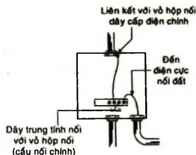
Hình 8-5. Liên kết vỏ hộp nối dây cấp điện chính
