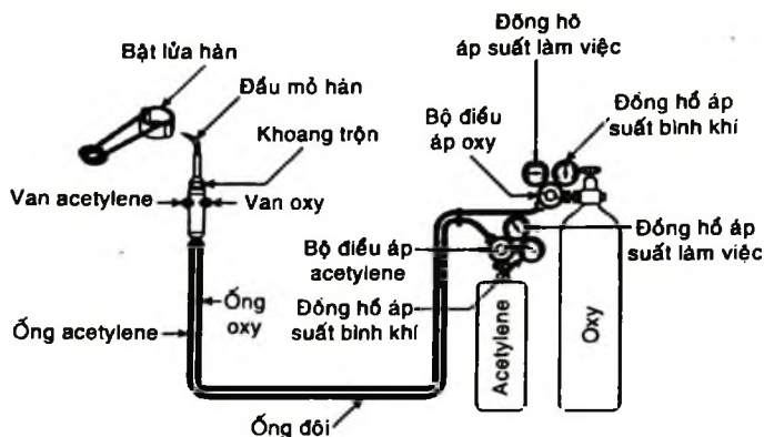
Hình 10-2. Thiết bị hàn oxyacetylene
