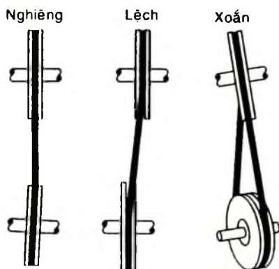
Hình 6-6. Các kiểu không thẳng hàng
