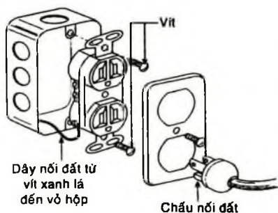
Hình 8-8. Cách liên kết ổ cắm điện
