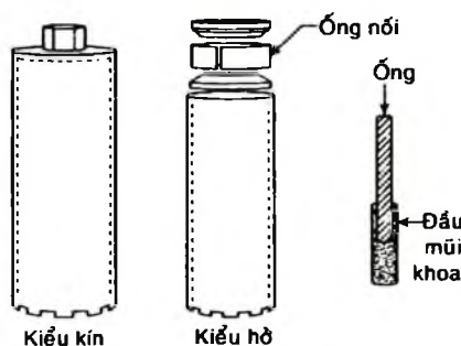
Hình 15-1. Mũi khoan lỗ kim cương.
