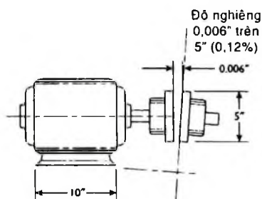
Hình 6-12. Các trục không thẳng hàng.
