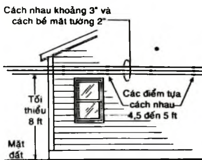
Hình 7-4. Dây cáp điện chạy trên bề mặt tường
