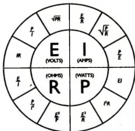
Hình 1-3. Mười hai công thức của định luật Watt.
