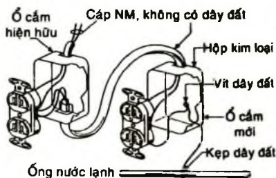
Hình 8-11. Phương pháp bổ sung ổ cắm nối đất vào nguồn không nối đất.
