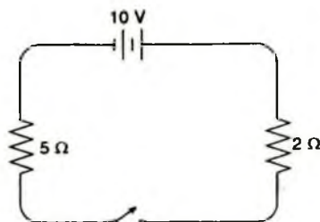
Hình 1-5. Mạch nối tiếp
