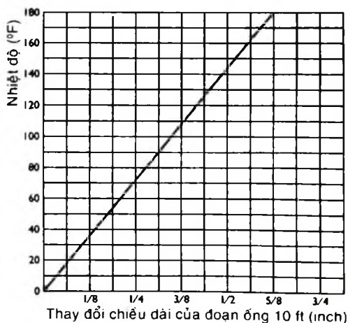
Hình 12-9. Sự giãn nở của ống luồn dây PVC
