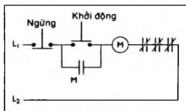
Hình 4-4. Mạch điều khiển.
