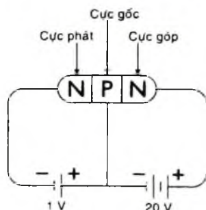
Hình 2-4. Transistor NPN được nối vào mạch điện
