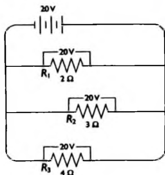
Hình 1-7. Mạch điện song song
