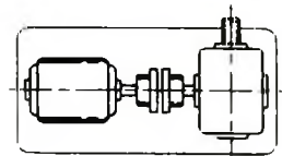
Chỉnh thẳng hàng theo chiều ngang Lấy các số đo theo mặt phẳng ngang, tại hai bên khớp nối
