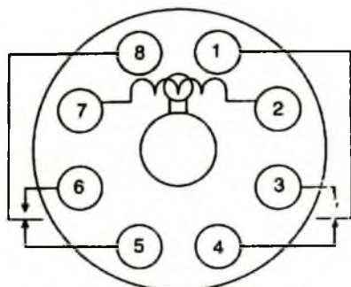
Hình 9-3. Rơ-le tám chân
