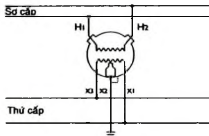
Hình 11-6. Nối kết công suất điện một pha
