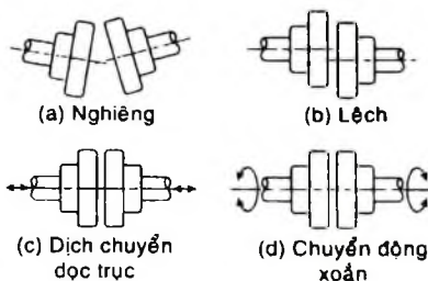
Hình 6-8. Các khớp mềm
