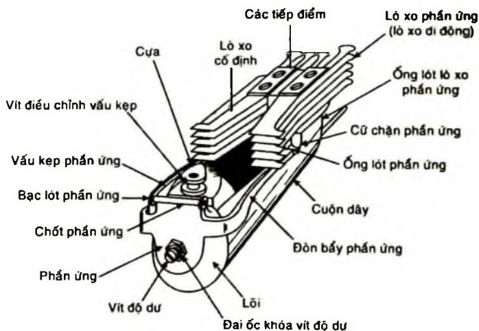
Hình 9-5. Cấu tạo rô-le.
