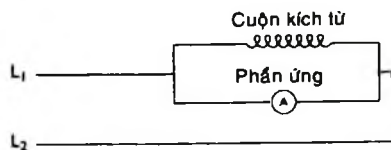
Hình 4-6. Động cơ dc mắc shunt (song song)
