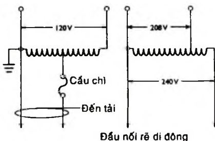
Hình 11-2. Biến áp tự ngẫu.
