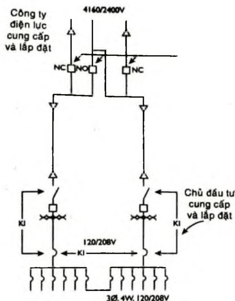
Hình 3-8. Sơ đồ hệ thống phân phối điện công nghiệp.
