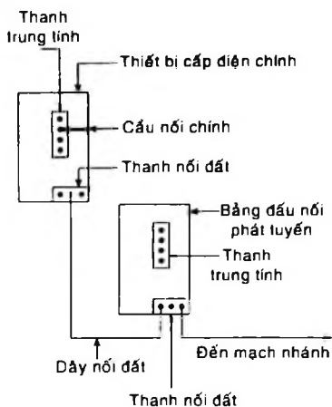
Hình 7-17. Nối đất bảng đấu nối phát tuyến
