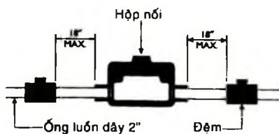
Hình 14-4. Các đệm kín xung quanh hộp nối
