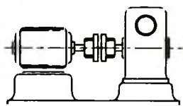
Chỉnh thẳng hàng theo chiều đứng Lấy các số đo theo mặt phẳng đứng, tại đỉnh và chân khớp nối
