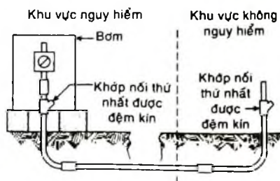
Hình 14-14. Xác định các khu vực nguy hiểm
