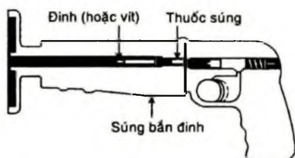
Hình 15-3. các bộ phận của súng bắn đinh.
