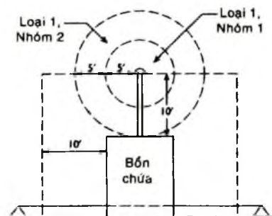
Hình 14-18. Các khu vực Loại 1 xung quanh bồn chứa
