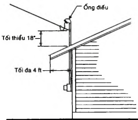
Hình 7-3. Cách lắp trụ dừng dây cấp điện chính.
