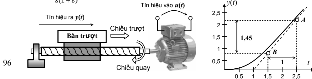
Hình 3.15: Đối tượng nhận dạng là động cơ chỉnh vị trí.
