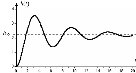
Hình 3.27: Hàm quá độ của đối tượng dao động bậc hai.
