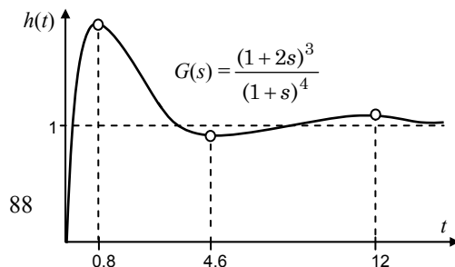
Hình 3.8: Hàm quá độ với 3 điểm cực trị.
