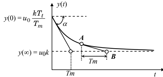
Hình 3.26: Xác định tham số cho mô hình Lead (dẫn qua).
