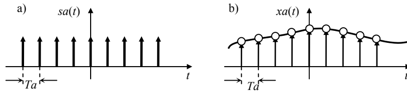
Hình 2.3: a) Đồ thị hàm răng lược. b) Mô hình hóa quá trình trích mẫu tín hiệu.
