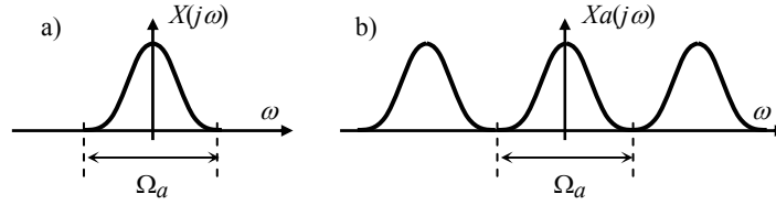
Hình 2.6: Giải thích định lý Shannon–Khatelnikov và chu kỳ trích mẫu của Nyquist.
