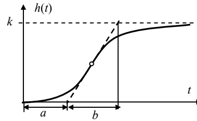
Hình 1.4: Xác định tham số cho mô hình đối tượng động cơ một chiều.
