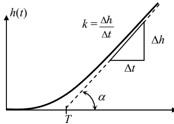
Hình 3.14: Hàm quá độ của khâu IT 1 .
