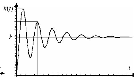
Hình 3.9: Dạng hàm quá độ có vô số điểm cực trị phân bố cách đều nhau trên và dưới đường giới hạn h(\infty) = k .
