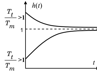
Hình 3.5: Hàm quá độ cho ví dụ 2.
