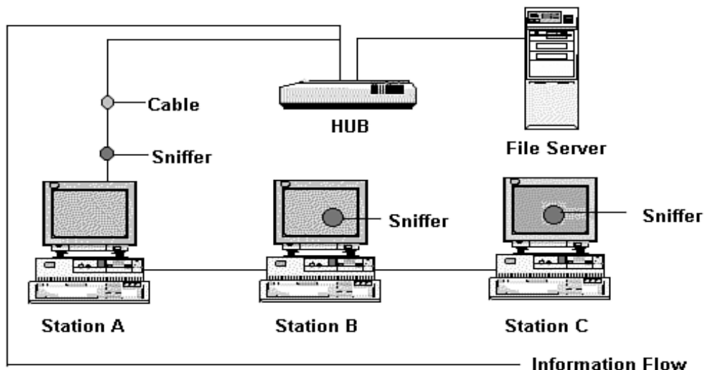
Hình 6.3: Các vị trí đặt sniffer trên 1 segment mạng
