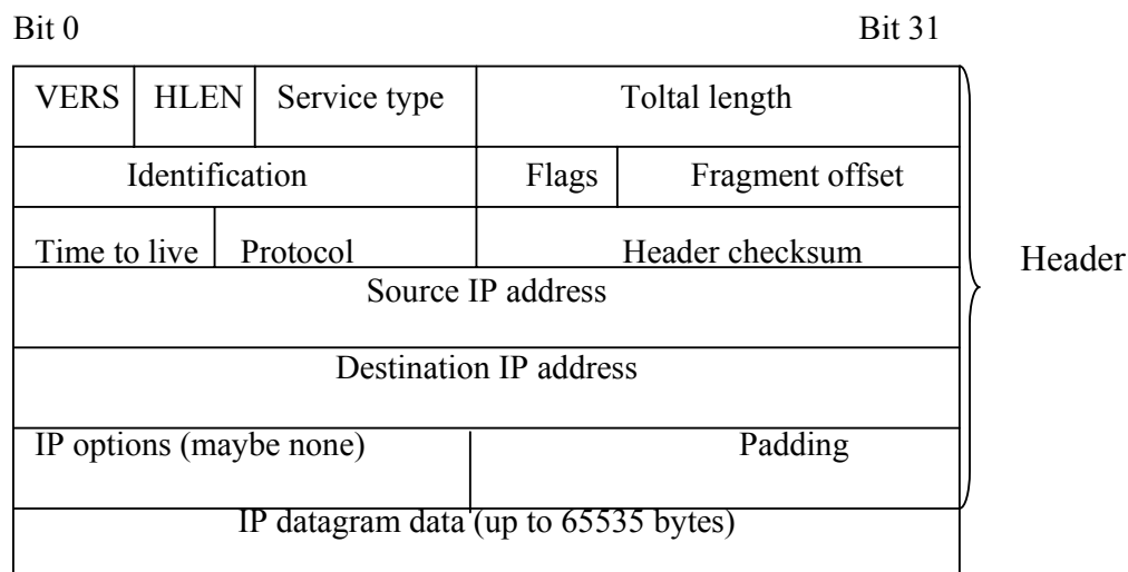
Hình 2.5: Cấu trúc gói dữ liệu TCPIP
