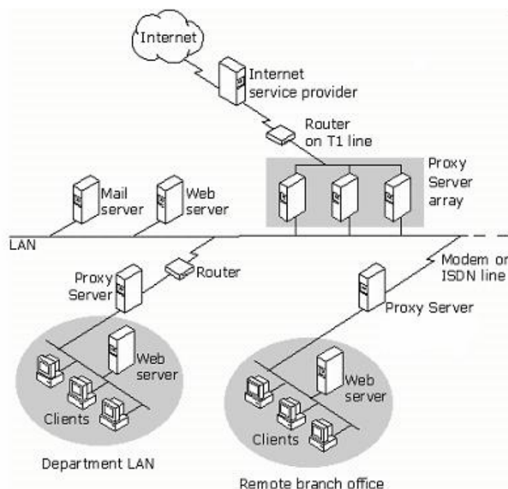
Hình 5.19: Mô hình kết nối mạng
