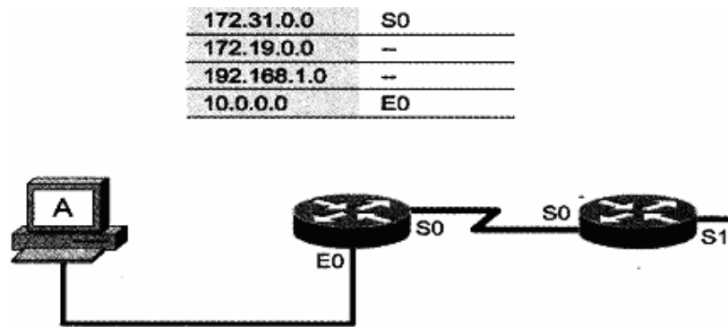
Hình 3.43: Sử dụng bảng định tuyến để truyền tải các gói tin
