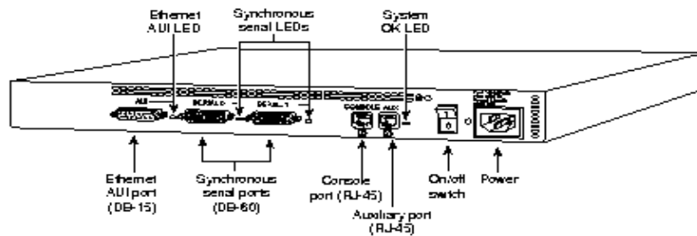
Hình 3.2: Bộ định tuyến Cisco 2501
