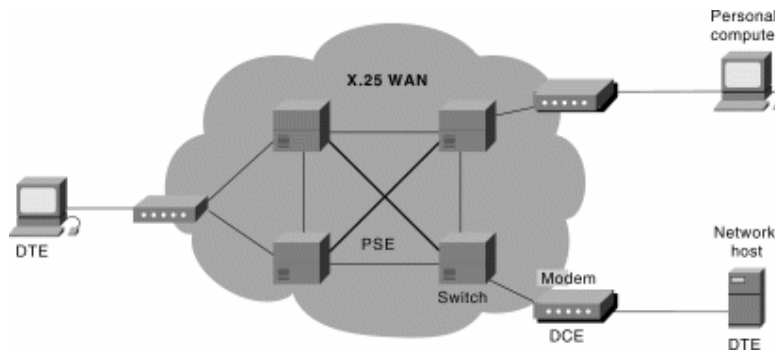
Hình 3.29: Mô hình kết nối X.25
