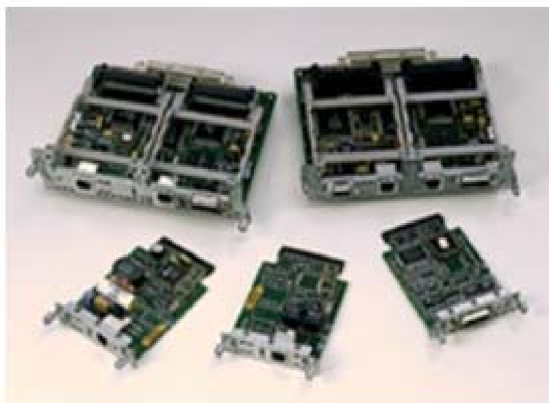
Hình 3.12: Module Ethernet có khe cắm WAN
