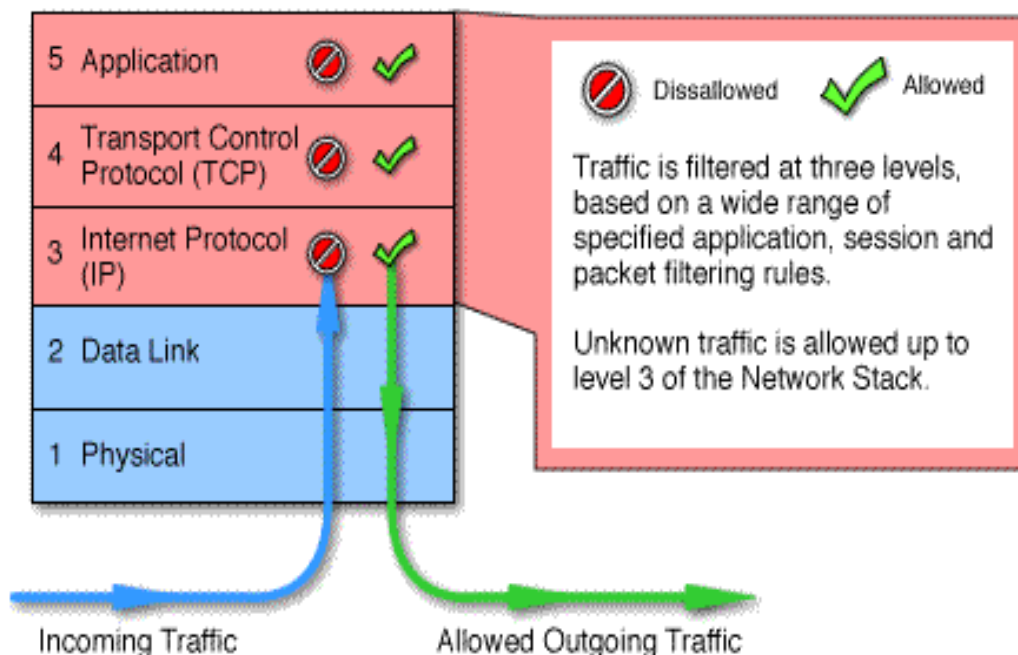
Hình 6.14: Stateful multilayer inspection firewall
