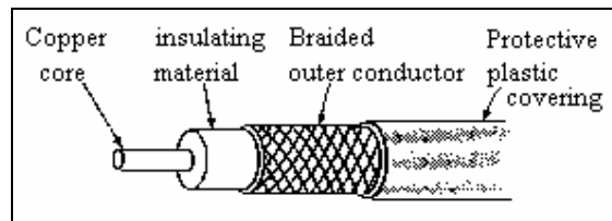
Hình 1.7. Cáp đồng trục
