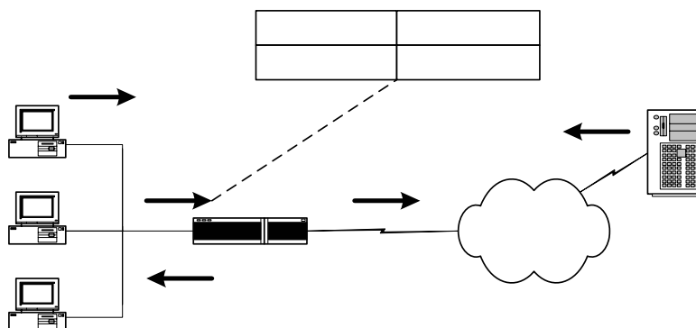
Hình 5.25: NAT
