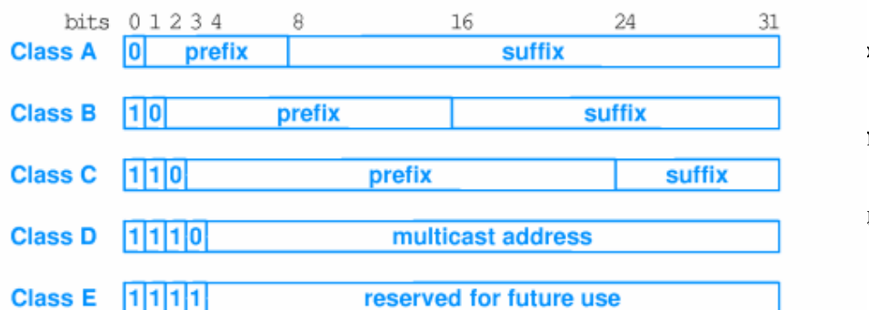
Hình 2.3: Cách đánh địa chỉ TCP/IP
