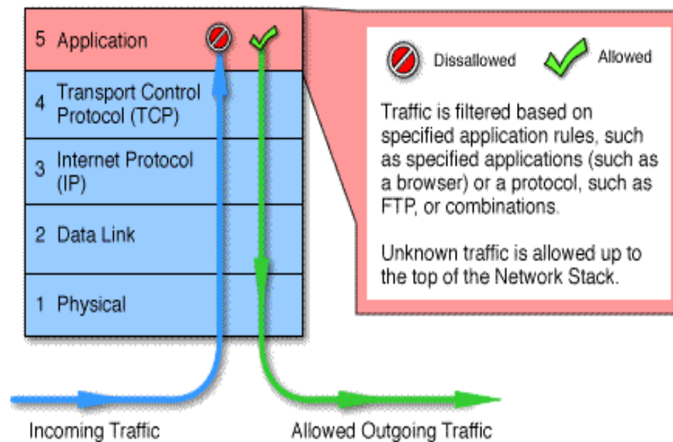
Hình 6.13: Application level gateway
