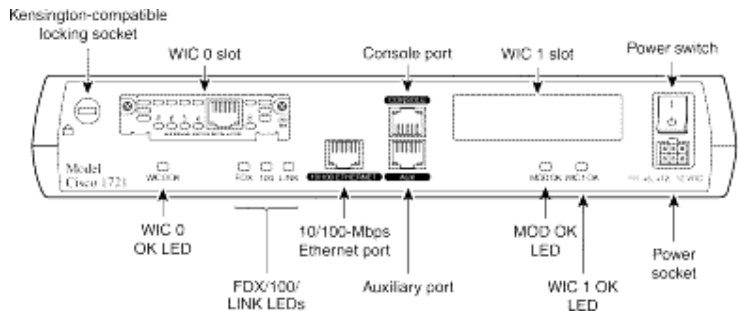
Hình 3.5: Bộ định tuyến Cisco 1721
