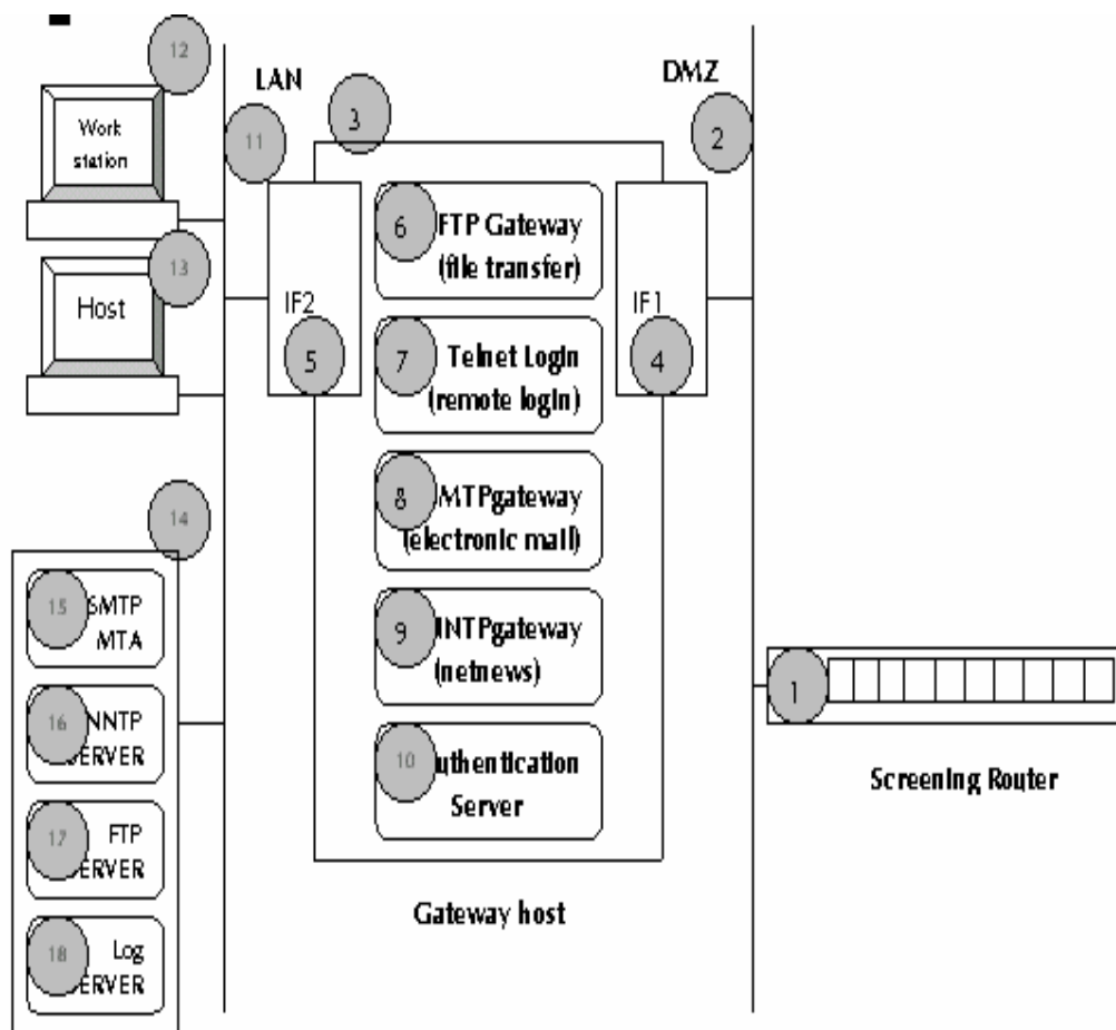
Hình 6.10: Các thành phần của hệ thống firewall
