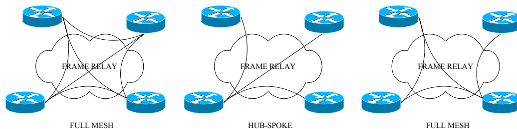
Hình 3.30: Mô hình kết nối Frame Relay
