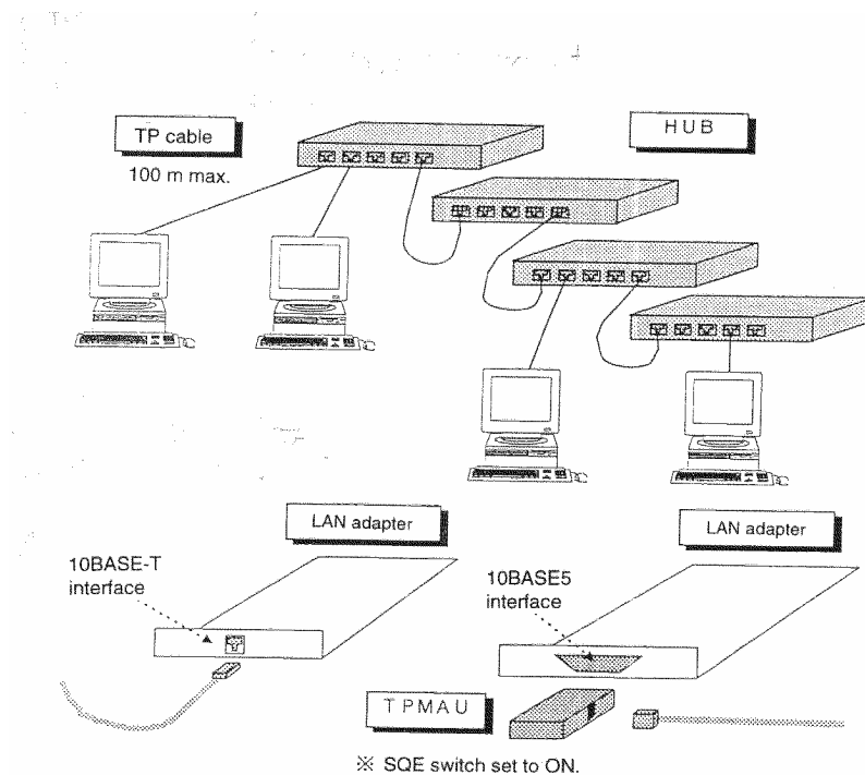
Hình 1.12: Nối mạng theo kiểu 10BASE-T với cáp UTP và HUB
