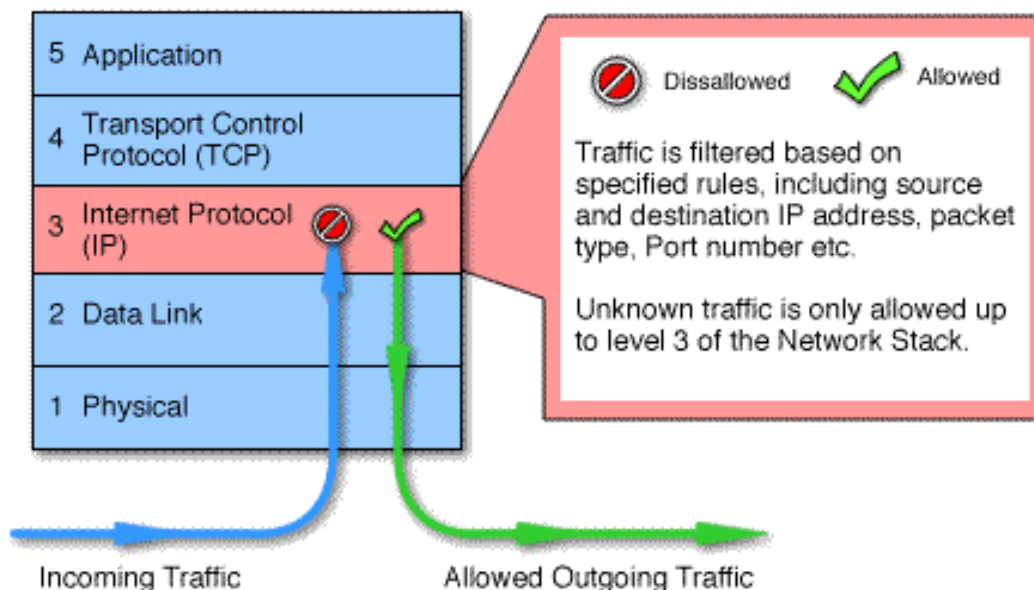
Hình 6.11: Packet filtering firewall
