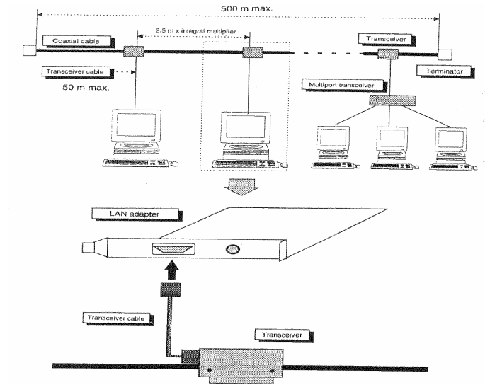
Hình 1.10. Kết nối theo chuẩn 10BASE5
