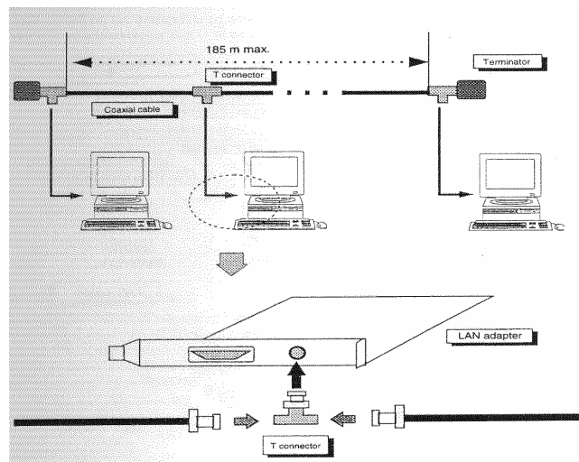
Hình 1.11: Nối theo chuẩn 10BASE2 với cáp đồng trục và đầu nối BNC
