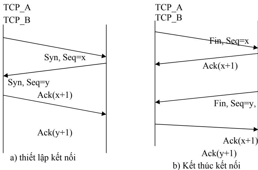
Hình 2.8: Quá trình kết nối theo 3 bước
