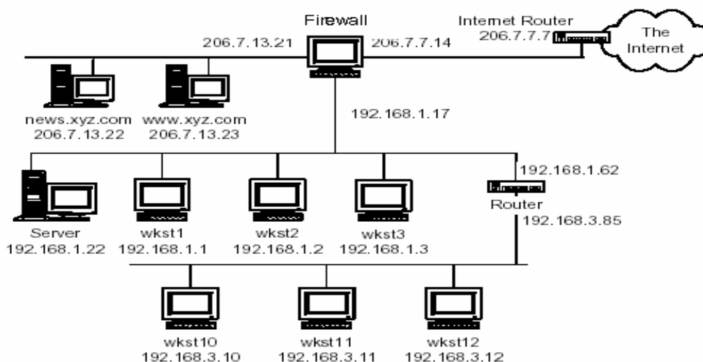
Hình 6.9: Kiến trúc hệ thống có firewall
