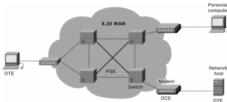
Hình 3.26: Chuyển mạch gói X.25
