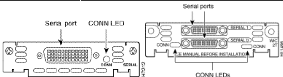
Hình 3.17: Card giao tiếp Serial
