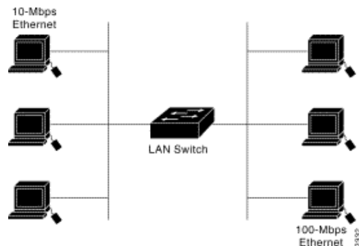
Hình 1.9. LAN Switch nối hai Segment mạng
